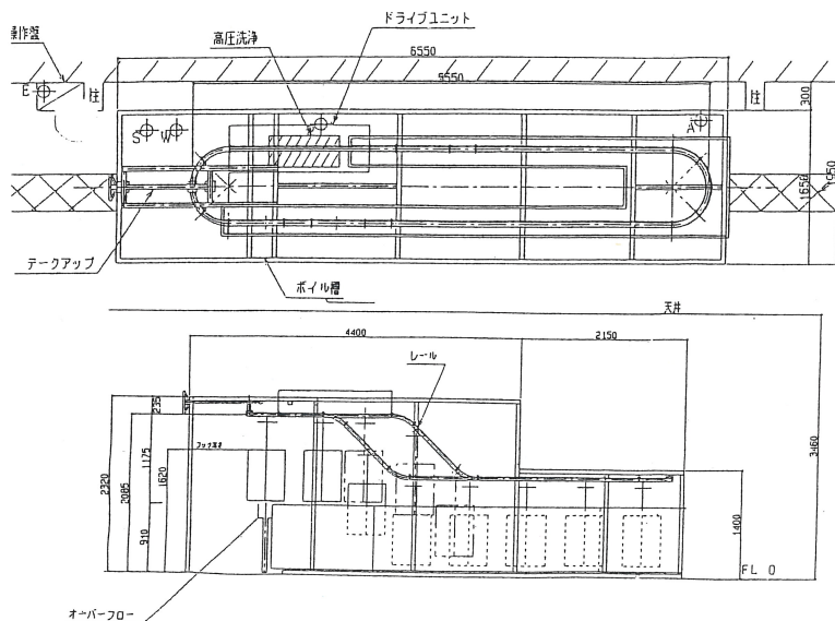
(本体平面、立面参考図)
