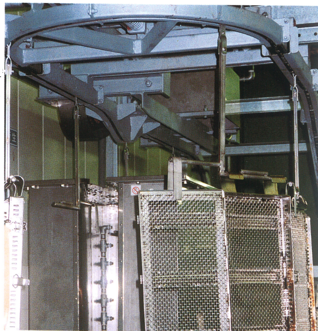
(本体横ハンガ吊り掛け部)
